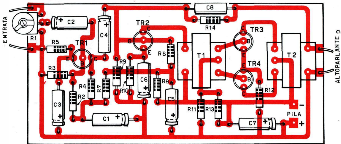
Fig. 8 - Nel caso volete costruire questo amplificatore su di una basetta di forma rettangolare anziché quadrata, non vi sarà difficile, seguendo i nostri suggerimenti, disegnare voi stessi il circuito stampato che potrà essere simile a questo da noi progettato. Raccomandiamo al lettore di controllare che i fori corrispondano con le dimensioni dei pezzi in modo da poterli correggere prima di incidere la piastrina.
