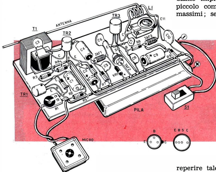
In figura è rappresentato lo schema pratico del radiomicrofono in dimensioni prossime a quelle reali del prototipo. Diremo anzi che per chiarezza di disegno, molti pezzi risultano occupare uno spazio di gran lunga superiore a quello realmente necessario; le dimensioni quindi risulteranno, dal lato pratico, anche inferiori.
