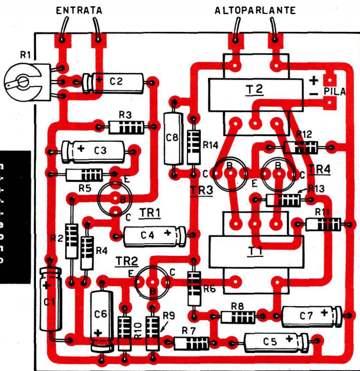
Fig. 6 - Procedendo ancora con questo semplice sistema noi possiamo arrivare a tracciare, per l'amplificatore sopra descritto, un circuito come quello indicato in questo disegno. Ricordiamo al lettore che percorsi di tracciato diverso dal circuito da noi disegnato non pregiudicano certo il funzionamento dell'amplificatore.
