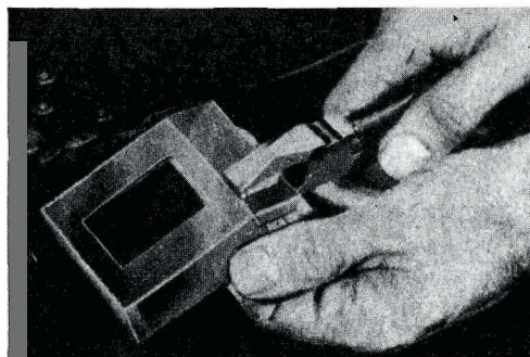
Fig. 5 - La scatola potrà essere costruita con sottili lamierino di zinco o di ottone, e per questo lavoro saranno sufficienti un paio di forbici, una pinza per piegare i bordi ed un saldatore per stagnare le giunture. Volendo la potrete costruire anche in legno o cartone.
